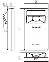
ECONAVI SENSOR (CZ-CENS1)
